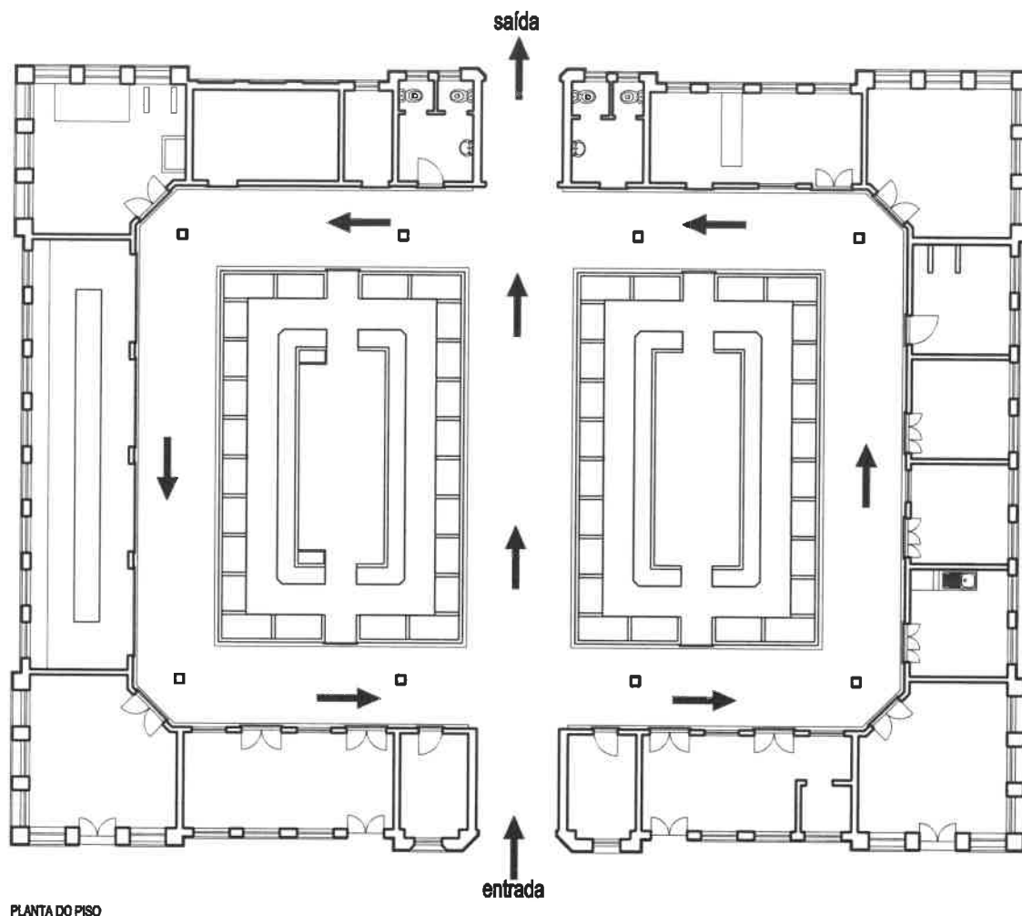
PLANTA DO PISO
